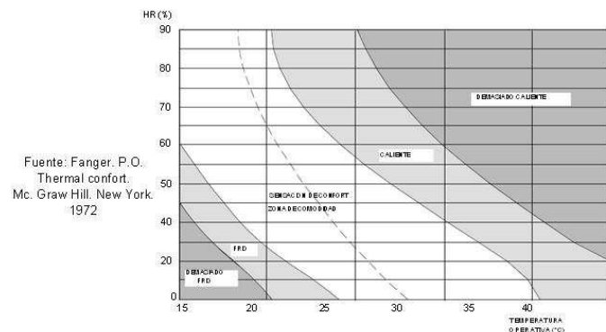
Fig. 4.6 Curva de confort (P.O. Fanger)
