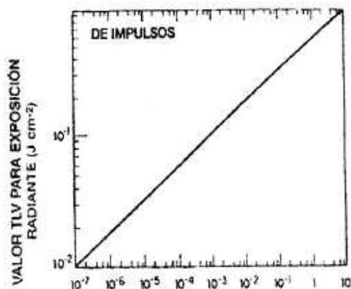
Figura 3 a. Valor TLV para exposición de la piel y los ojos a láser para radiación infrarroja lejana. (Longitudes de onda superiores a 1,4\ \mu m ).
