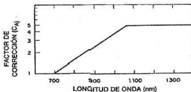
Figura 1. Factor de corrección de los valores TLV para \lambda = 700-1400 \text{ nm}^*
